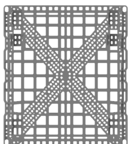
Vue du plateau à roues d'en haut
